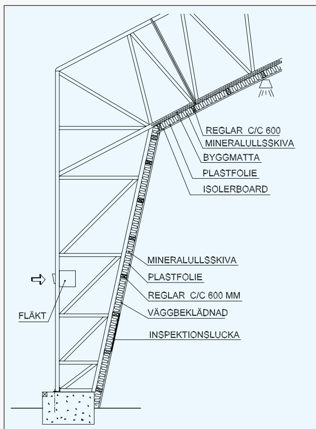
Principritning på isolering av PMH Thermohall.
